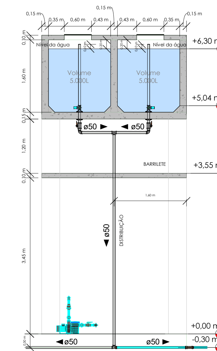
CORTE EE
