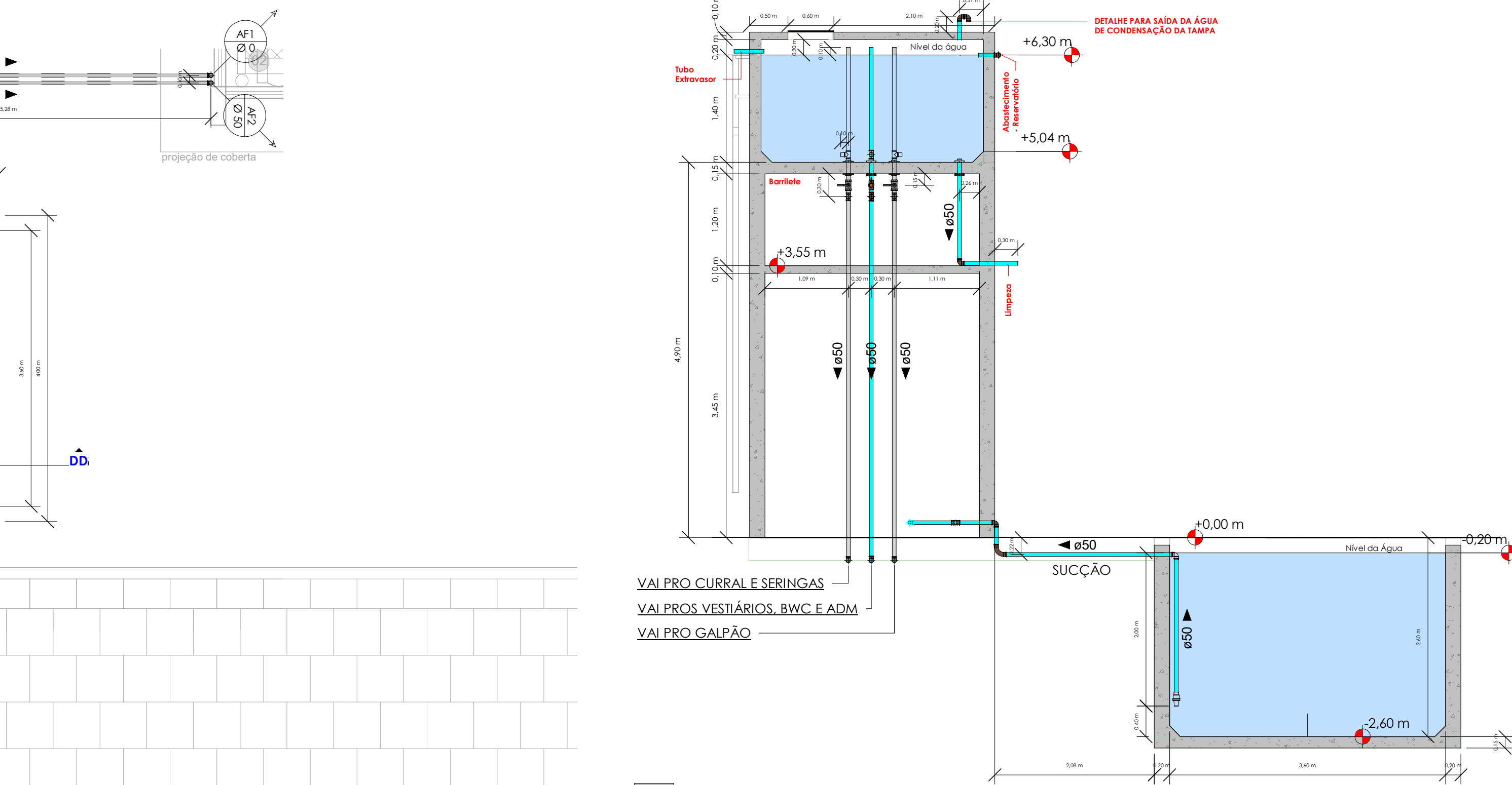
CORTE DD
