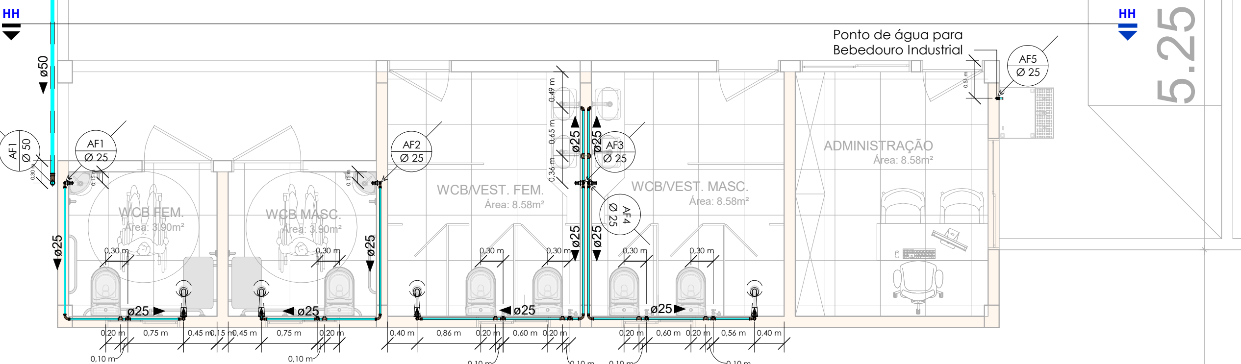
PLANTA BAIXA _BWC'S_VESTIÁRIOS_ADM - ESC
